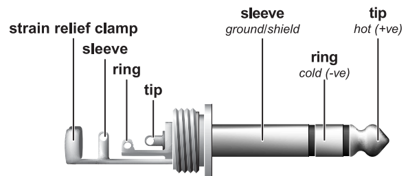
Fig. 6.4: 1/4" stereo plug
