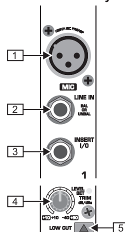
Fig. 2.1: Conexiones y reguladores de las entradas Mic / Line
