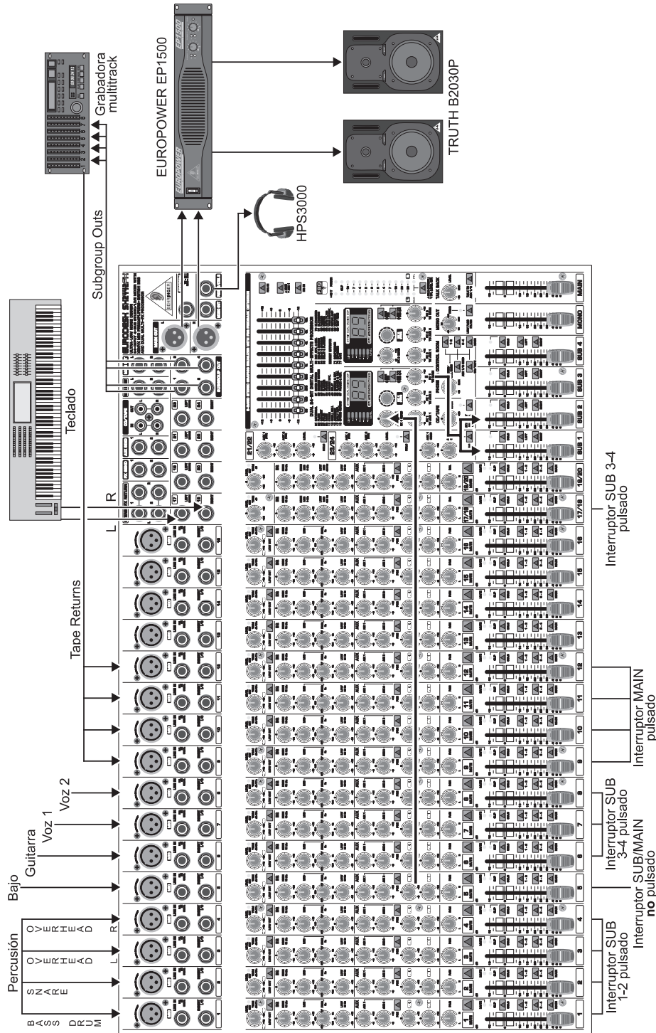
Fig. 4.1: Cableado de la mesa de mezclas para estudio
