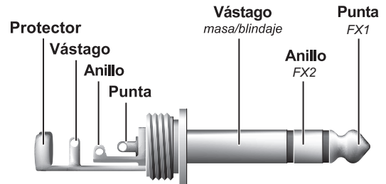
Fig. 5.5: Jack stereo de 6,3 mm para pedal
