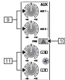
Fig. 2.3: Regulador AUX/FX Send en los canales
