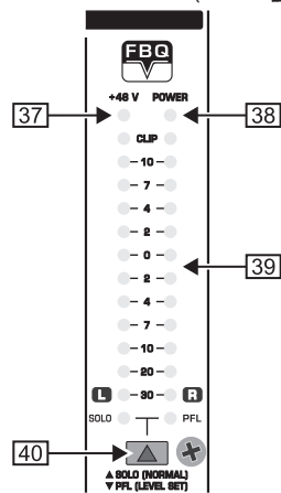
Fig. 2.16: Visualización de nivel
