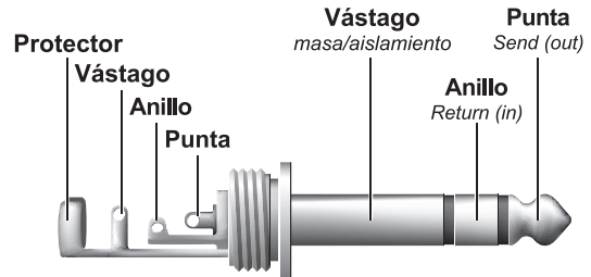
Fig. 5.7: Jack estéreo para envío y retorno de inserción
