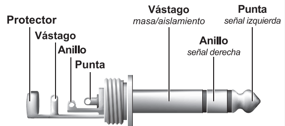
Fig. 5.6: Jack de 6,3 mm para auriculares
