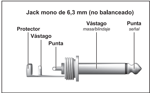
Fig. 5.1: Jack macho mono de 6,3 mm
