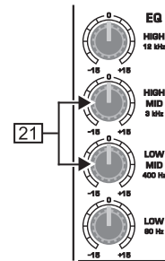
Fig. 2.6: Ecuador de los canales estéreo
