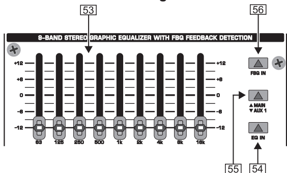
Fig. 2.24: Ecuador estereo gráfico
