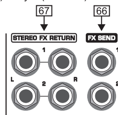
Fig. 2.26: Conexiones de envío y retorno de efectos
