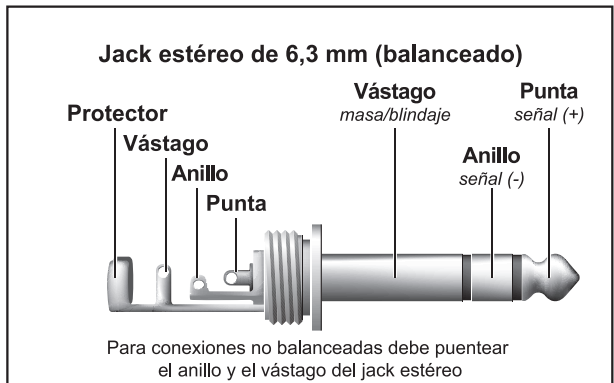
Fig. 5.2: Jack macho estéreo de 6,3 mm
