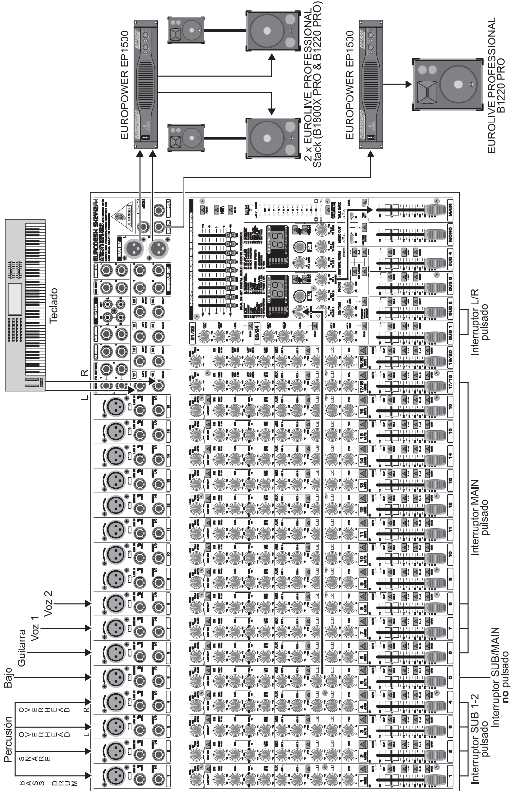
Fig. 4.2: Cableado de la mesa de mezclas para directo
